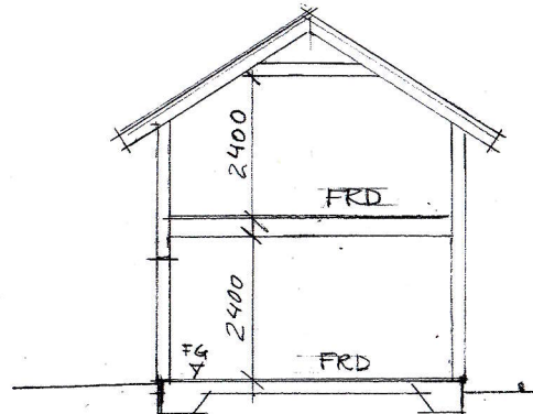
SEKTION A-A
